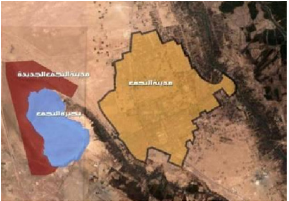
الشكل (12) موقع بحر النجف الذي يمكن استخدامه كخزان مائي
