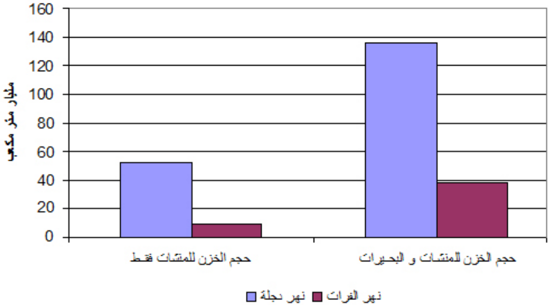
الشكل (10) حجم الخزن المائي للمتنشات ألقامه و البحيرات على النهرين
